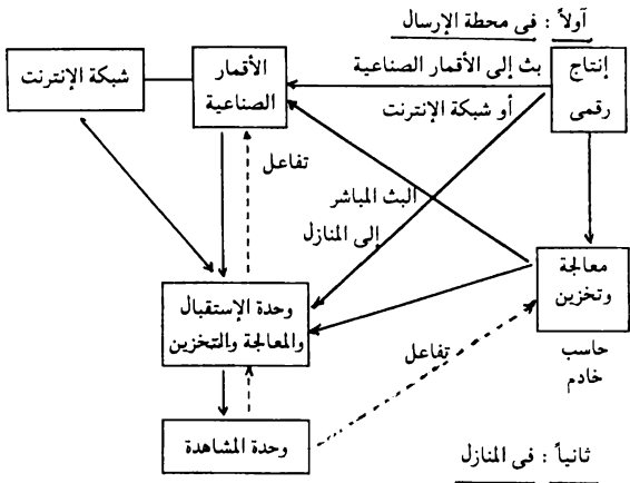
شكل رقم (٢١) البث والإستقبال فى التليفزيون التفاعلى
